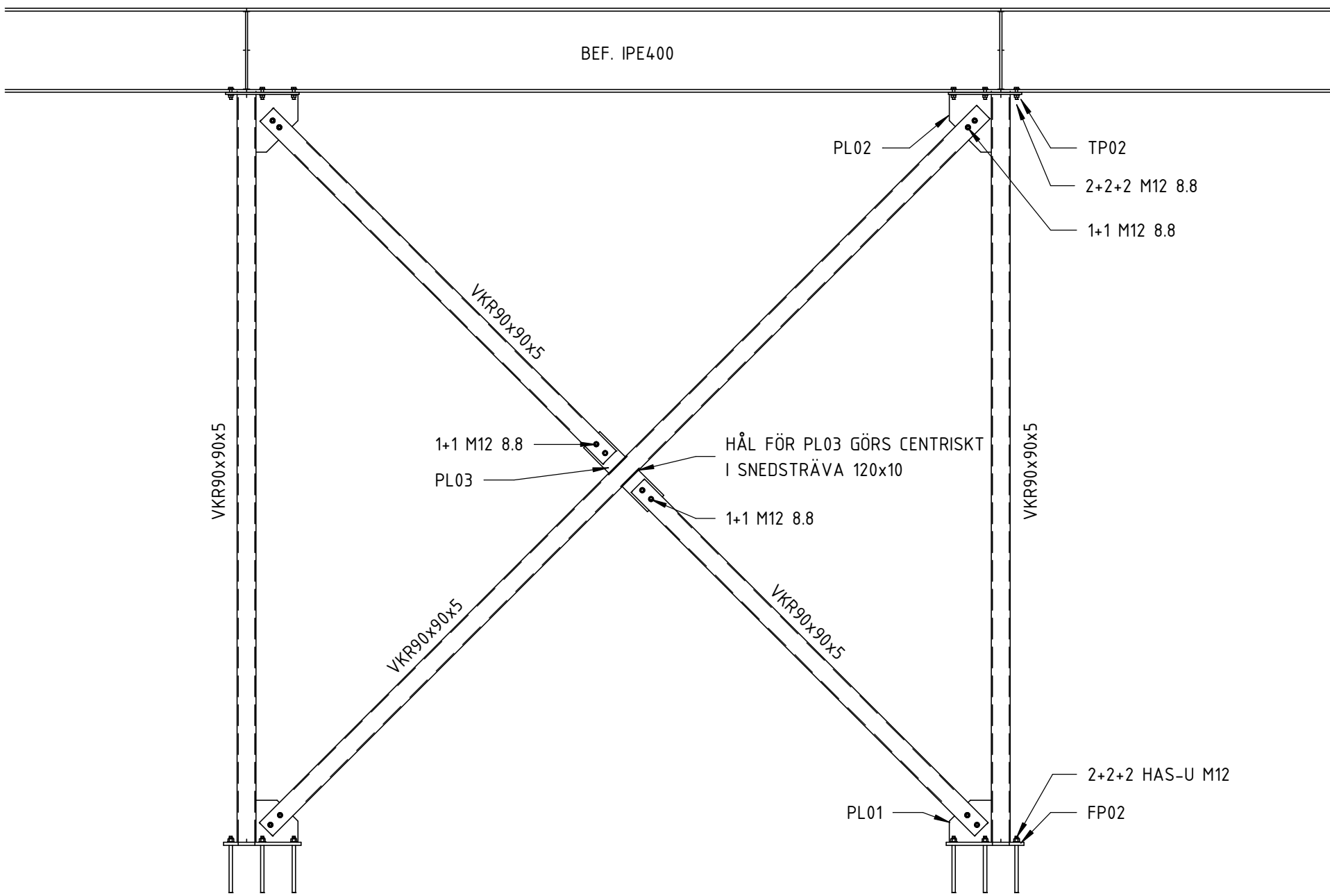
A241 1 : 25
